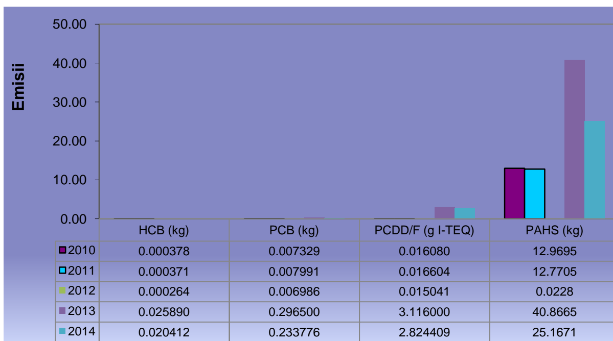
Fig. I.3.20. Evoluția emisiilor de poluanți organici persistenti, în perioada 2010 - 2014
