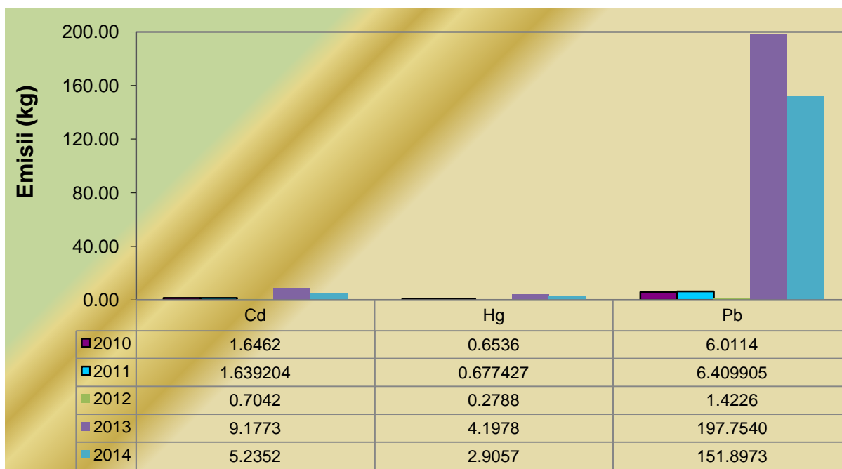
Fig. I.3.17. Evoluția emisiilor de metale grele din sectorul de activitate energie, în perioada 2010 - 2014
