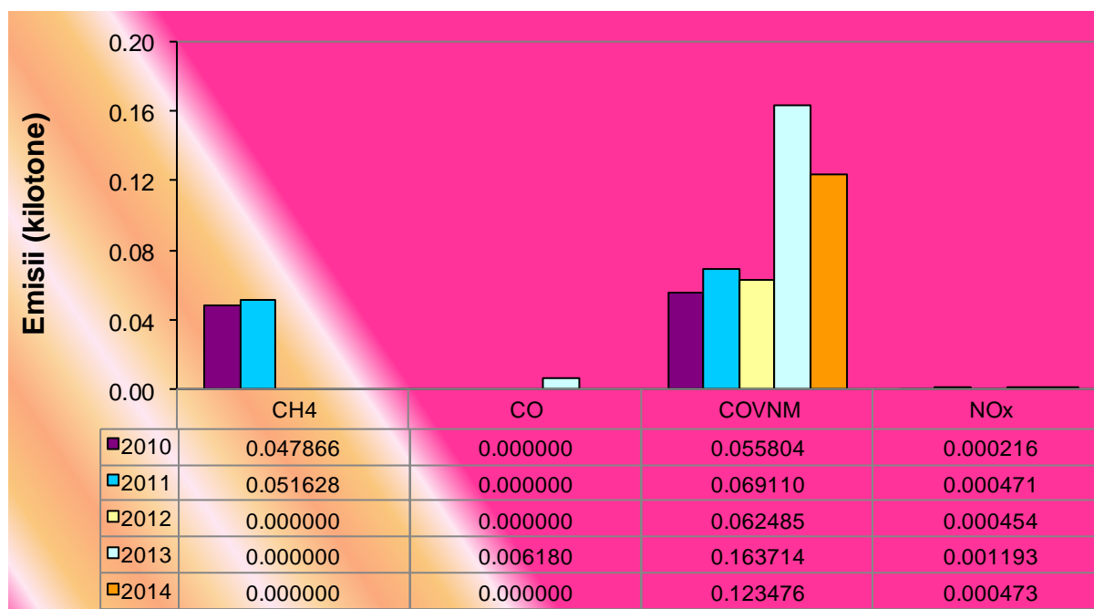
Fig. I.3.10. Evoluția emisiilor de precursori ai ozonului din agricultură, în perioada 2010 - 2014
