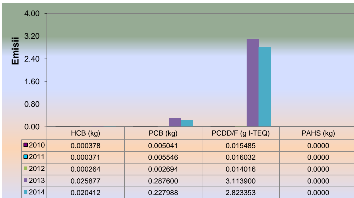
Fig. I.3.21. Evoluția emisiilor de poluanți organici persistenti din sectorul de activitate energie, în perioada 2010 - 2014
