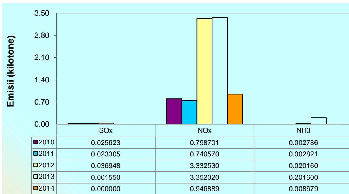
Fig. I.3.4. Evoluția emisiilor de substanțe acidifiante din transporturi, în perioada 2010 - 2014
