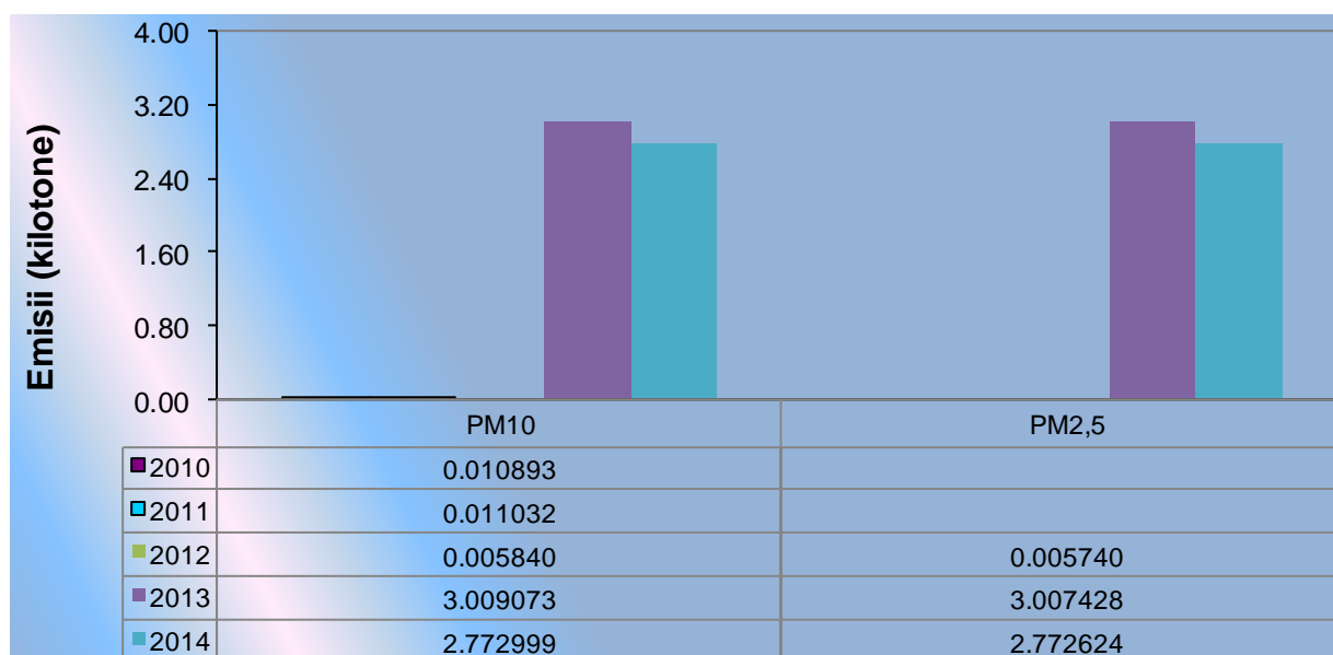
Fig. I.3.12. Evoluția emisiilor de particule primare din sectorul de activitate energie, în perioada 2010 - 2014
