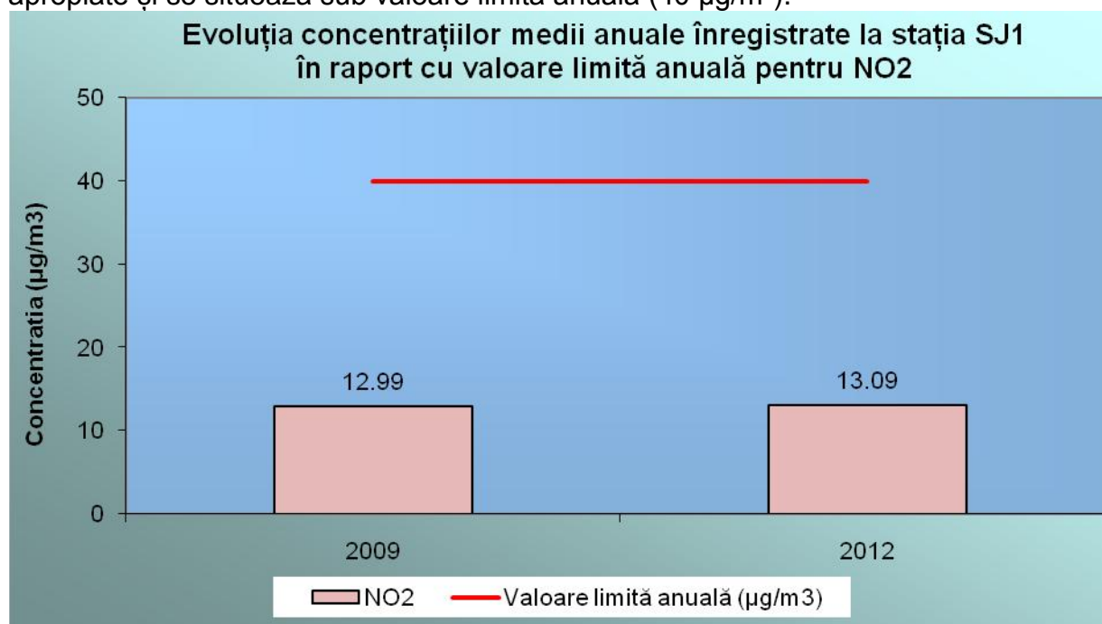
Fig. I.1.7. Evoluția concentrațiilor medii anuale pentru \text{NO}_2
