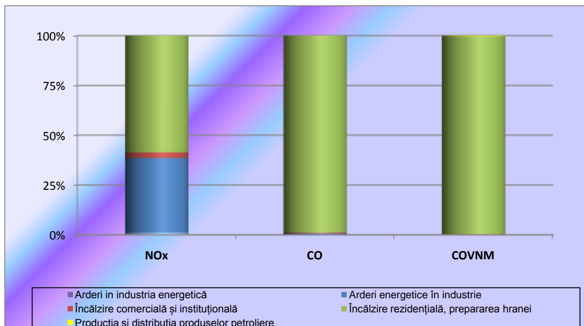
Fig. I.2.2. Ponderea emisiilor de precursori ai ozonului, pe sectoare de activitate din energie
