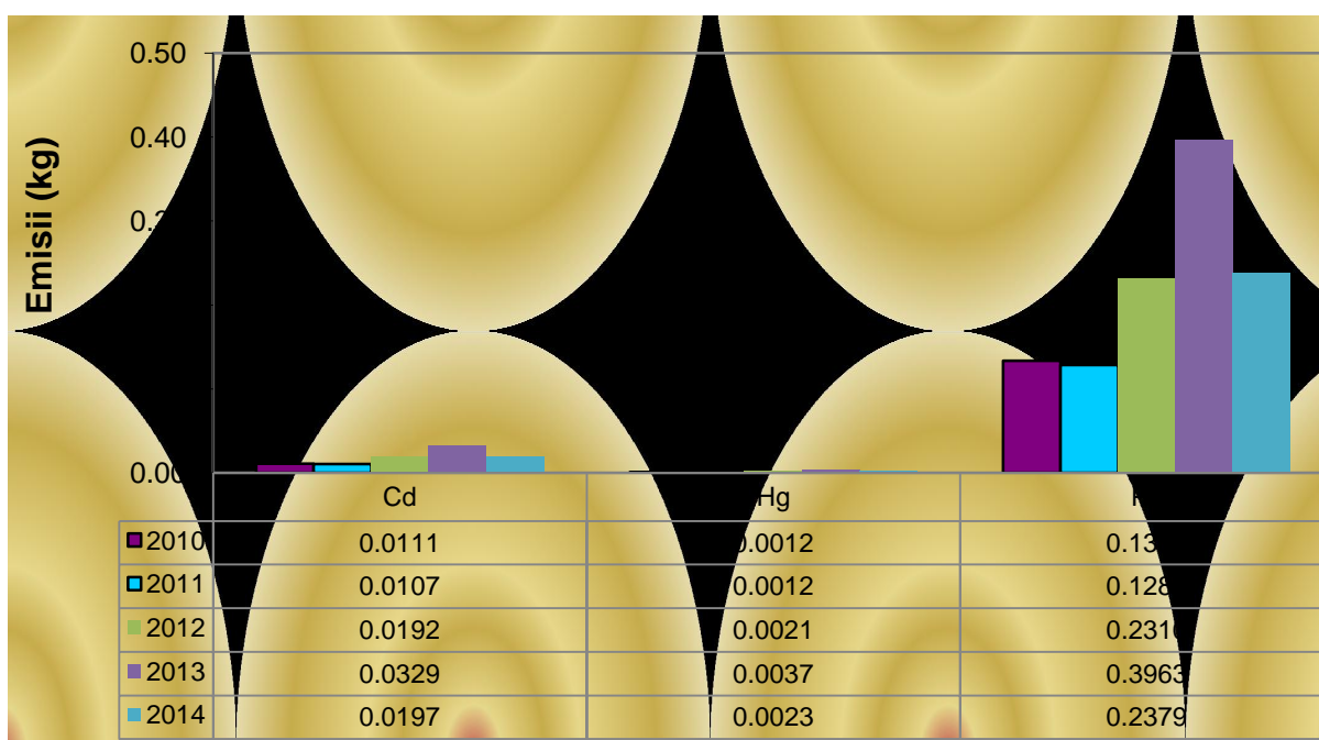
Fig. I.3.18. Evoluția emisiilor de metale grele din industrie, în perioada 2010 - 2014
