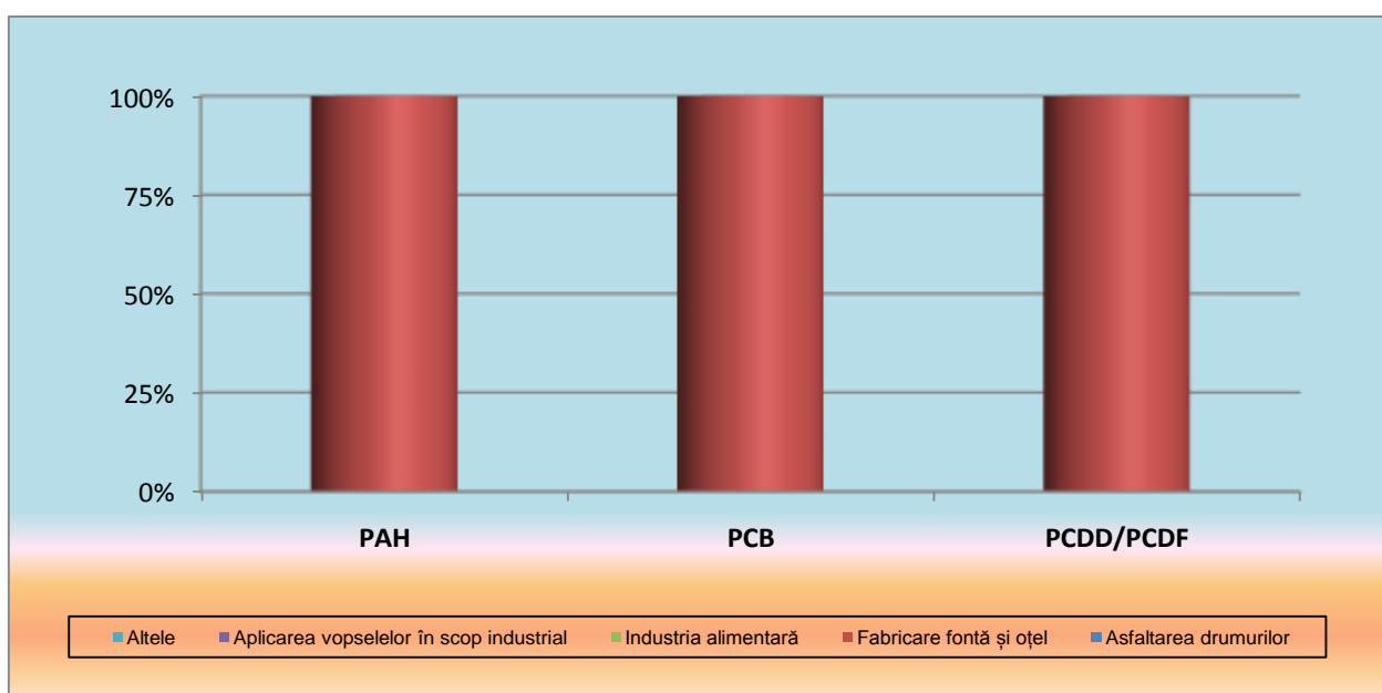
Fig. I.2.10. Ponderea emisiilor de poluanți organici persistenti pe sectoare de activitate din industrie
