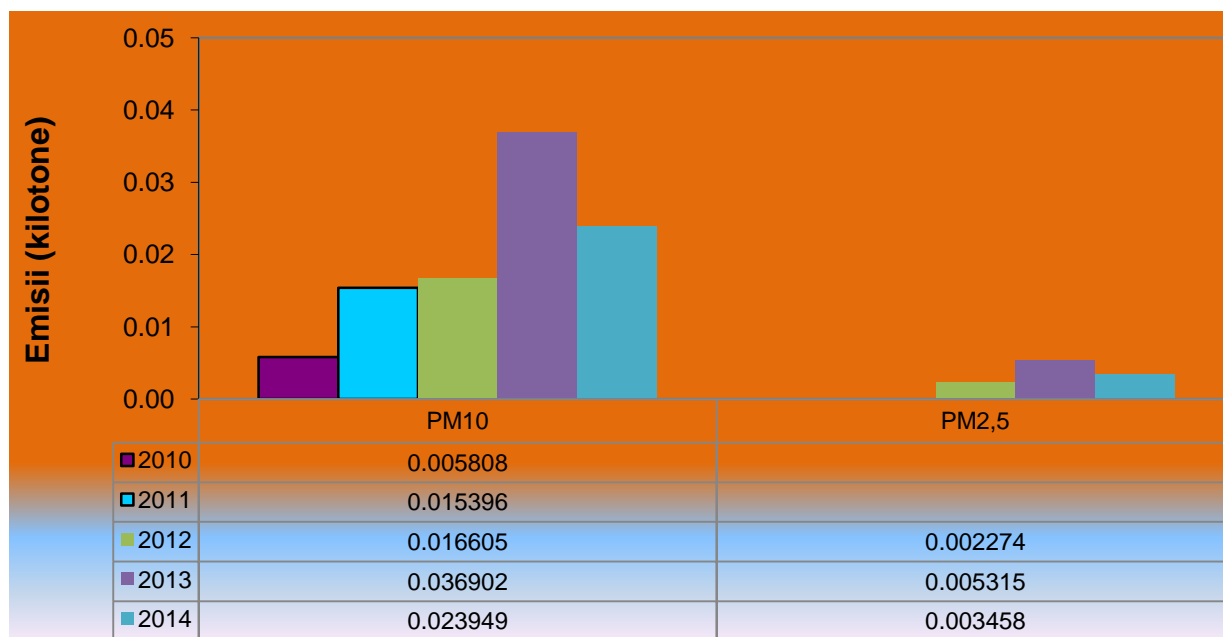
Fig. I.3.15. Evoluția emisiilor de particule primare din agricultură, în perioada 2010 - 2014
