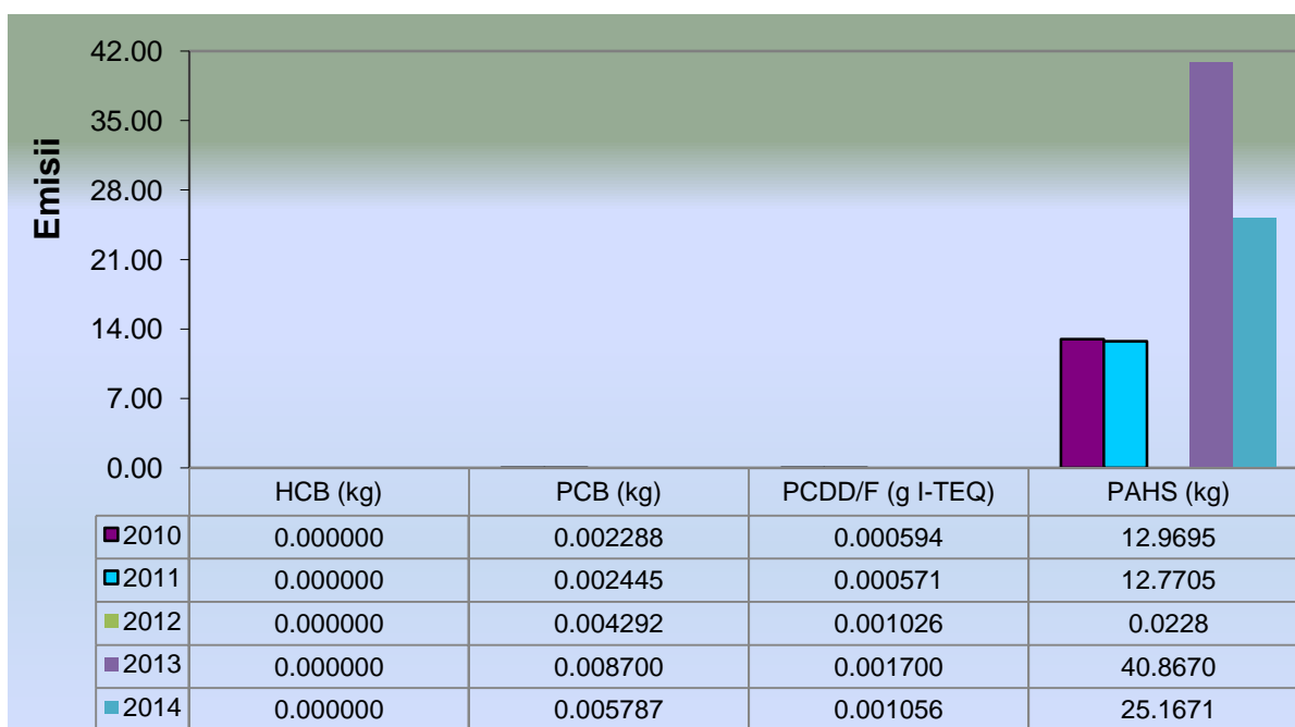
Fig. I.3.22. Evoluția emisiilor de poluanți organici persistenti din industrie, în perioada 2010 - 2014
