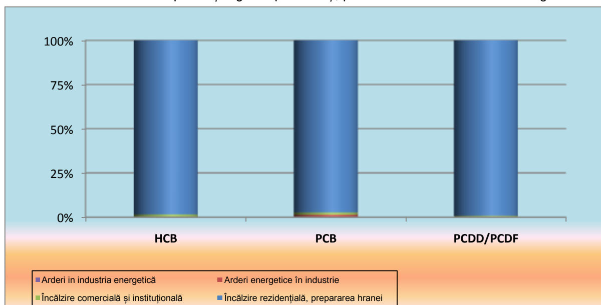
Fig. I.2.5. Ponderea emisiilor de poluanți organici persistenti pe sectoare de activitate din energie
