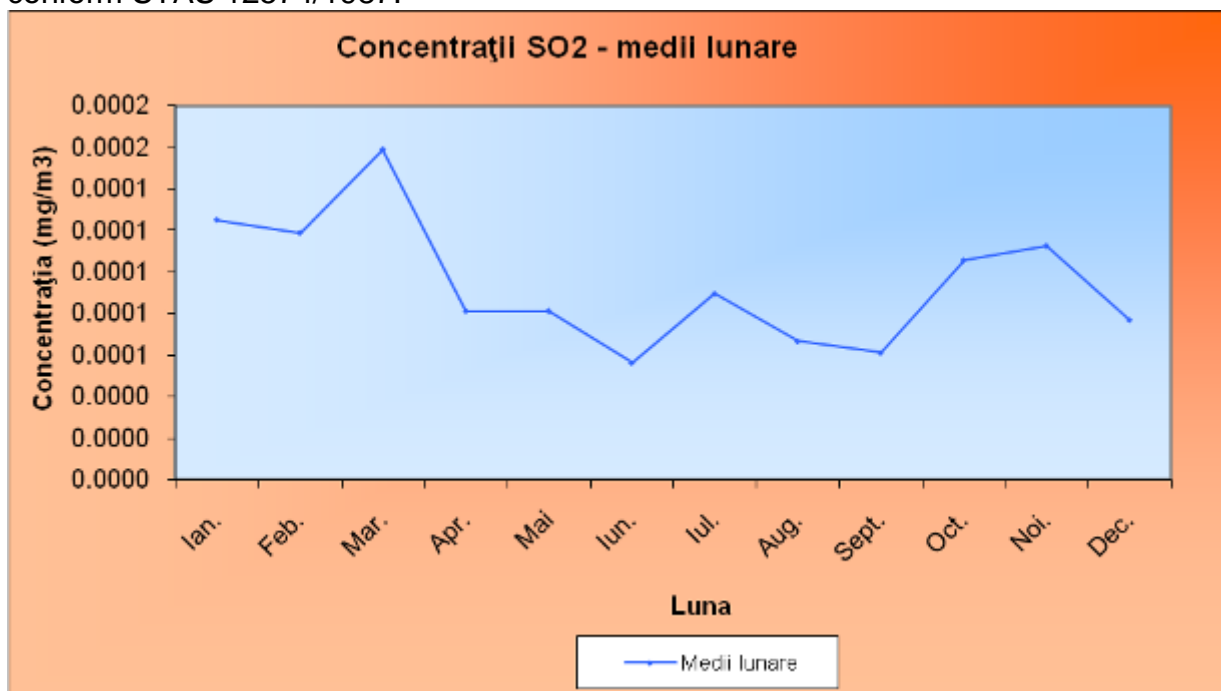
Fig. I.1.3. Concentrații de SO 2 – medii lunare
