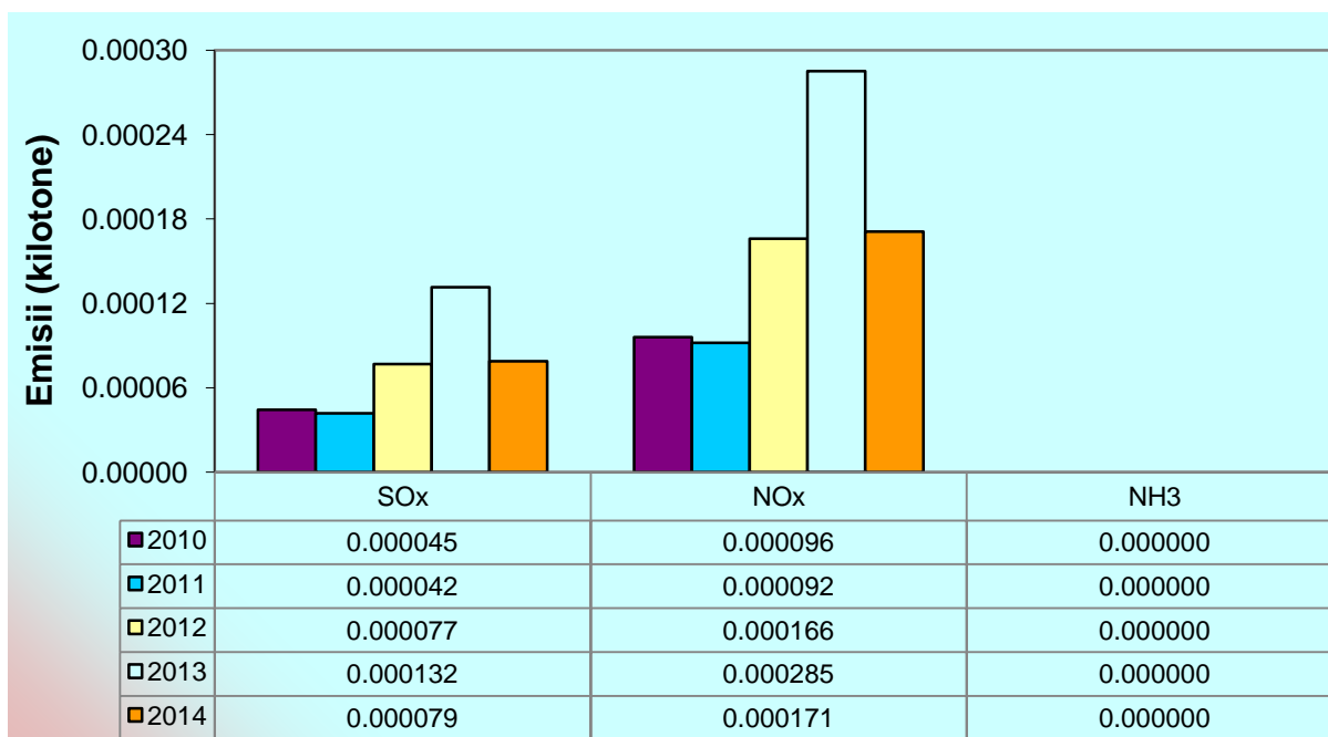
Fig. I.3.3. Evoluția emisiilor de substanțe acidifiante din industrie, în perioada 2010 - 2014
