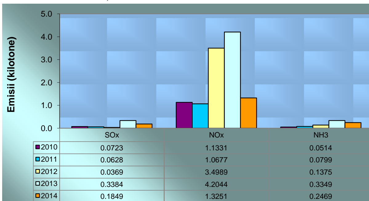
Fig. I.3.1. Evoluția emisiilor de substanțe acidifiante în perioada 2010 - 2014
