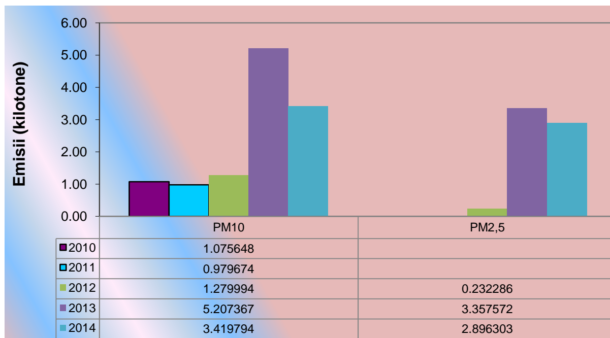
Fig. I.3.11. Evoluția emisiilor de particule primare, în perioada 2010 - 2014
