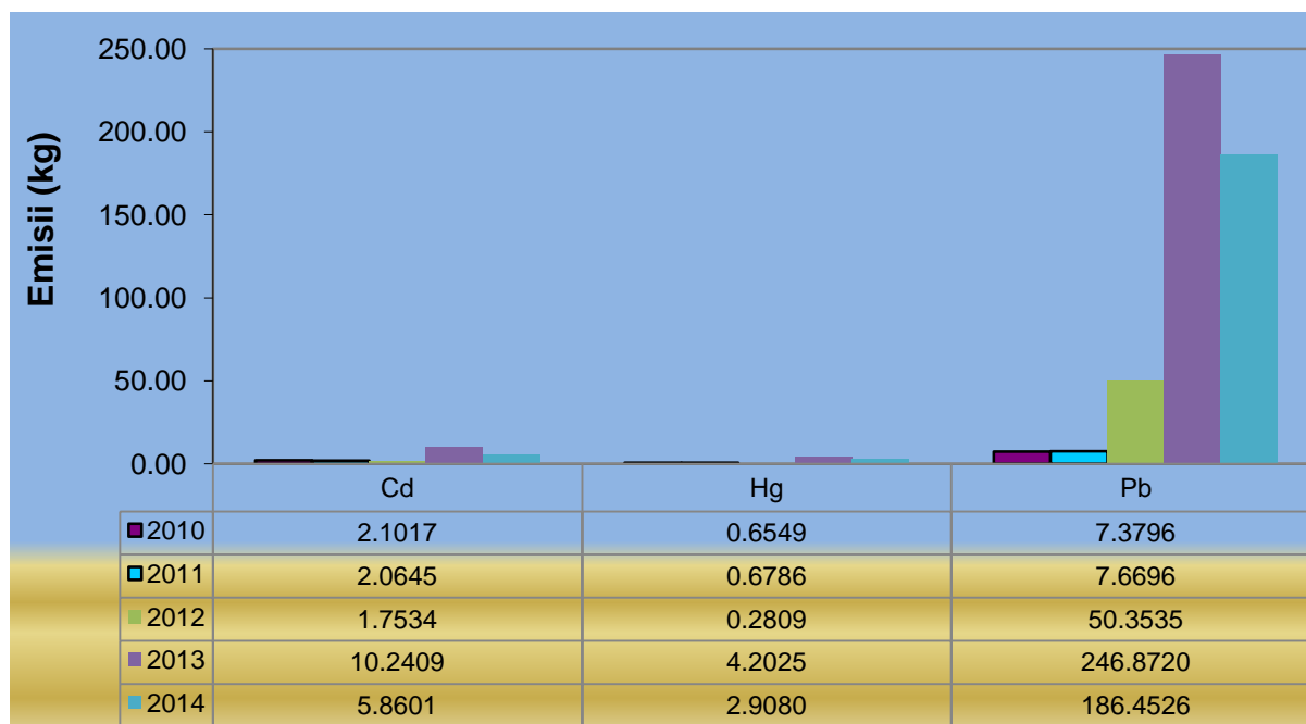
Fig. I.3.16. Evoluția emisiilor de metale grele, în perioada 2010 - 2014
