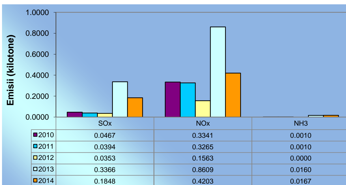
Fig. I.3.2. Evoluția emisiilor de substanțe acidifiante din sectorul de activitate energie, în perioada 2010 - 2014
