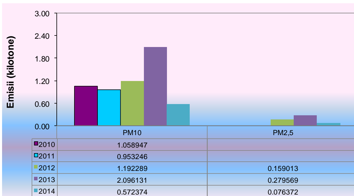
Fig. I.3.13. Evoluția emisiilor de particule primare din industrie, în perioada 2010 - 2014
