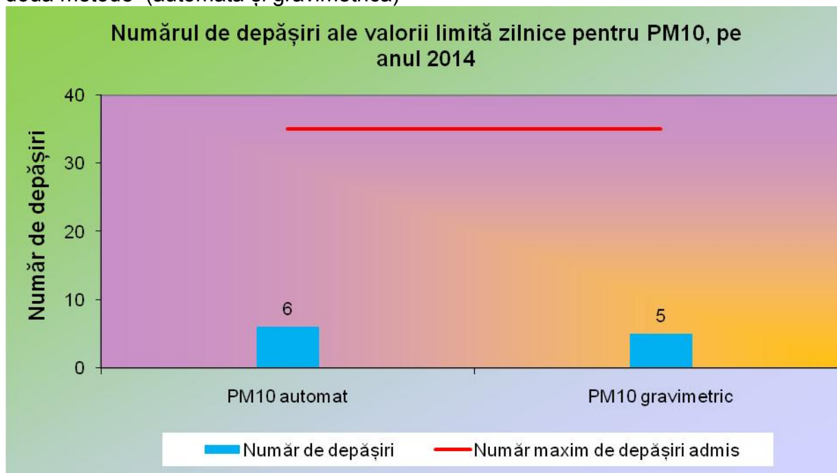
Fig. I.1.12. Numărul de depășiri a valorii limită zilnice pentru PM10
