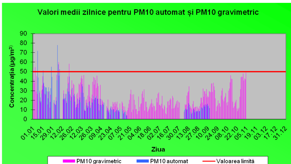
Fig. I.1.4. Valorile ale mediilor zilnice pentru pulberi în suspensie
