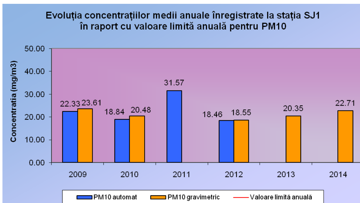
Fig. I.1.11. Evoluția mediilor anuale pentru PM10 automat și PM10 gravimetric
