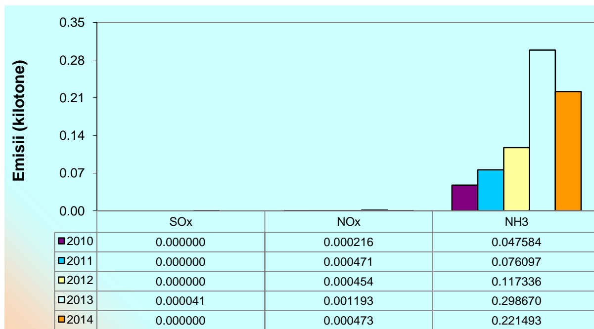
Fig. I.3.5. Evoluția emisiilor de substanțe acidifiante din agricultură, în perioada 2010 - 2014
