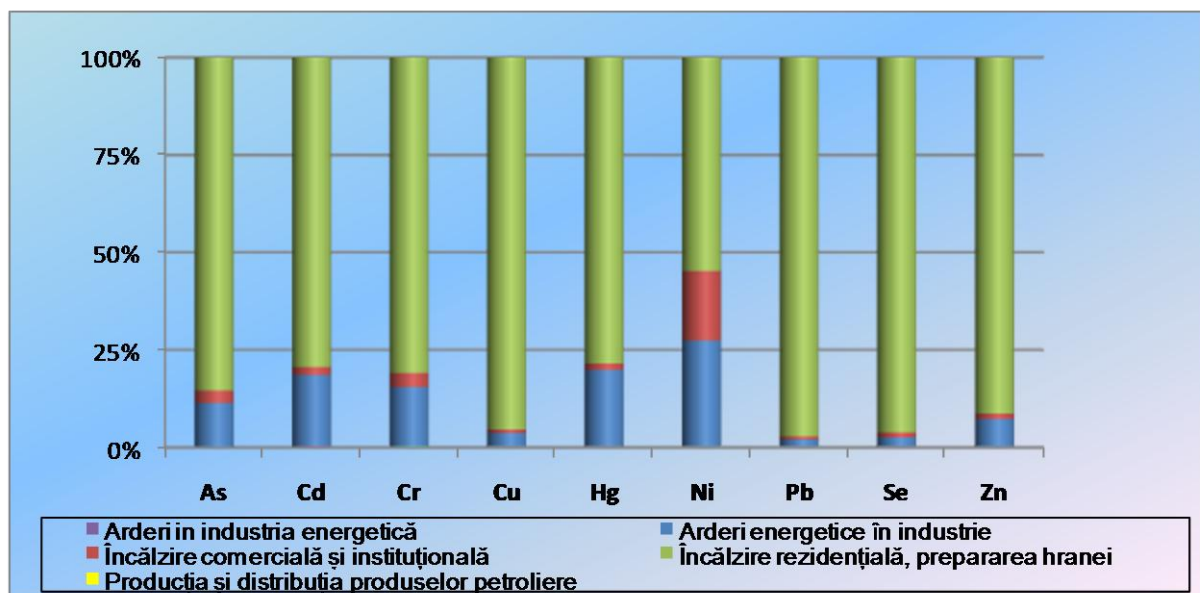
Fig. I.2.4 Ponderea emisiilor de metale grele pe sectoare de activitate din energie
