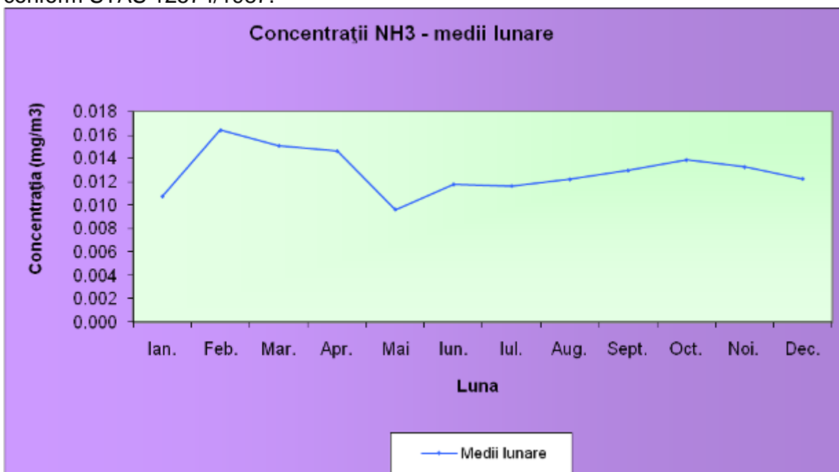
Fig. I.1.6. Concentrații de NH 3 – medii lunare
