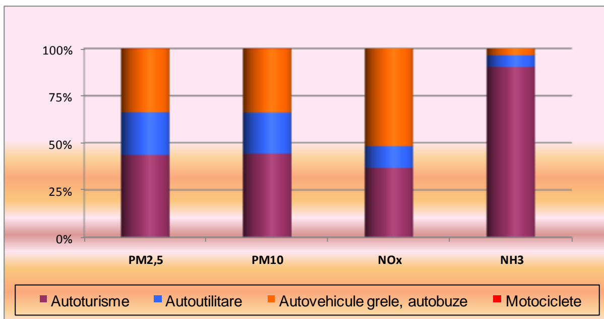
Fig. I.2.13. Ponderea emisiilor de particule prim. și precursori secund. de particule pe tipuri de vehicule de transport
