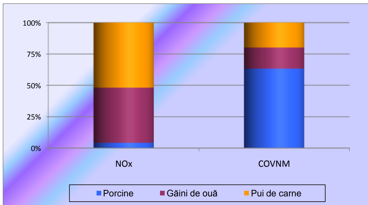
Fig. I.2.16. Ponderea emisiilor de precursori ai ozonului, pe sectoare de activitate din agricultură
