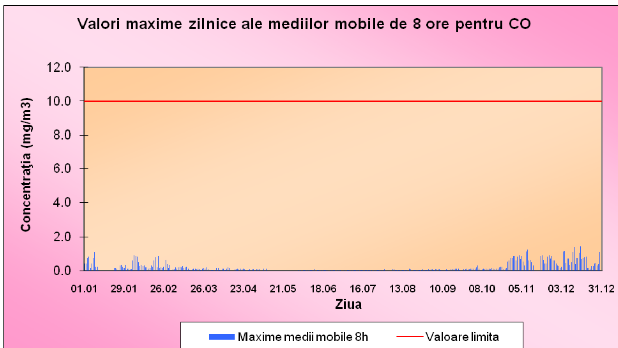
Fig. I.1.5. Valorile maxime zilnice ale mediilor mobile de 8 ore pentru poluantul CO
