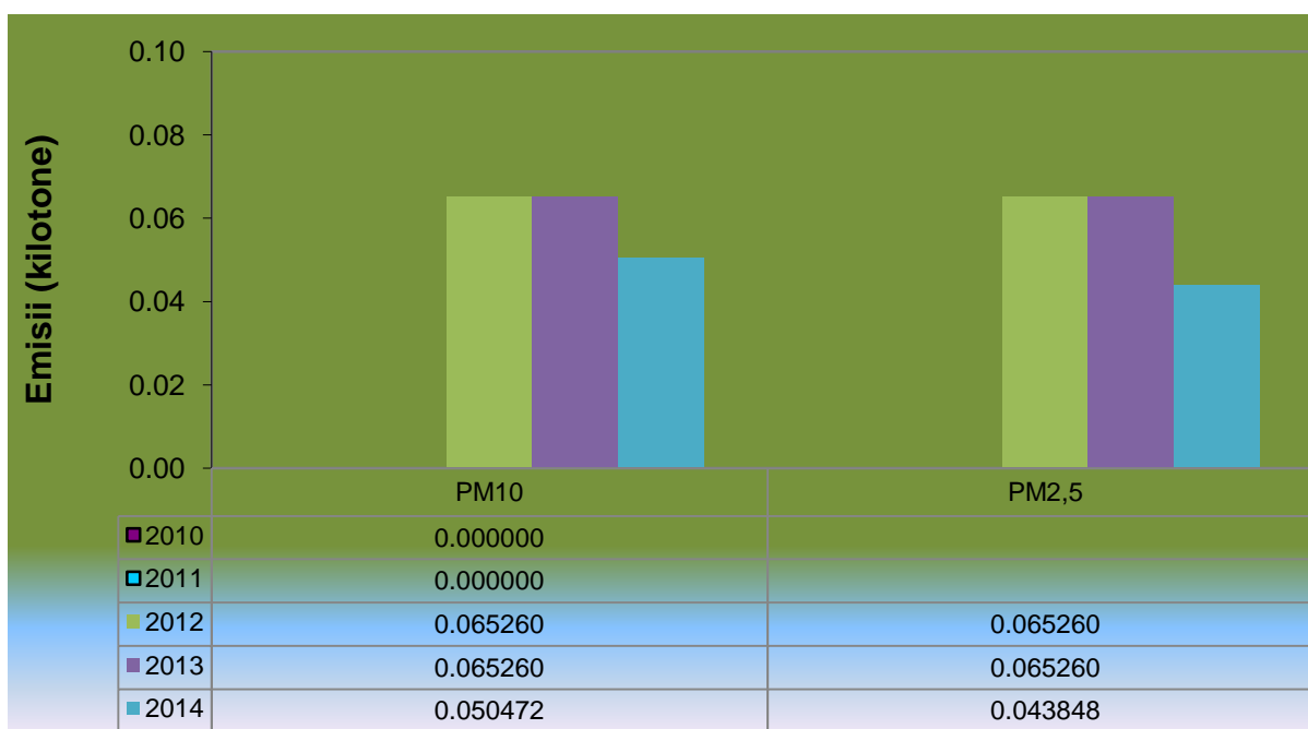
Fig. I.3.14. Evoluția emisiilor de particule primare din transporturi, în perioada 2010 - 2014
