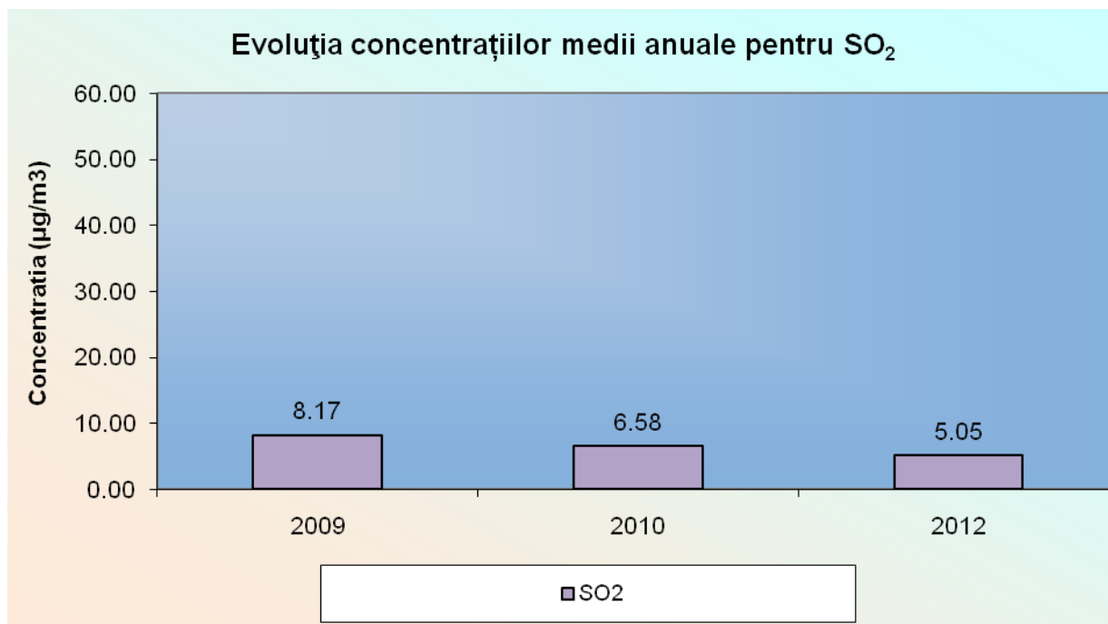
Fig. I.1.8. Evoluția concentrațiilor medii anuale pentru SO 2
