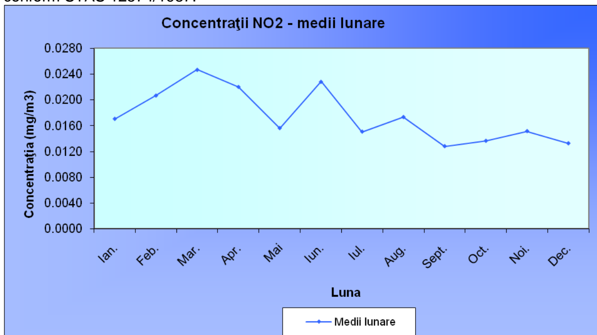
Fig. I.1.2. Concentrații de NO 2 – medii lunare
