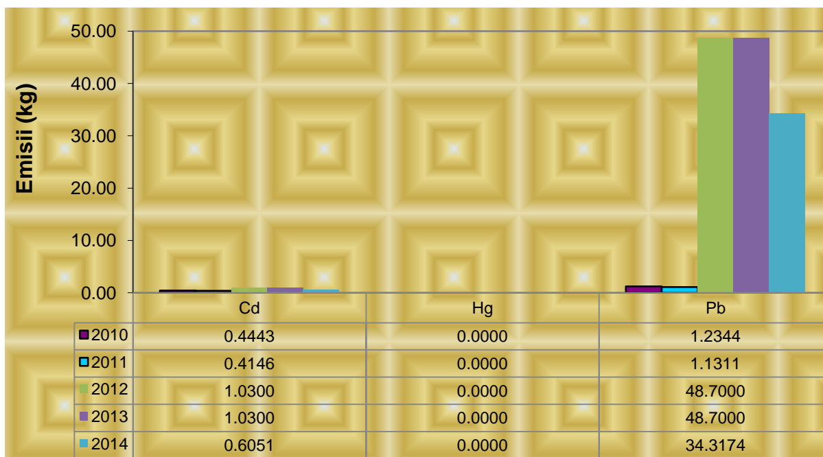
Fig. I.3.19. Evoluția emisiilor de metale grele din transport, în perioada 2010 - 2014
