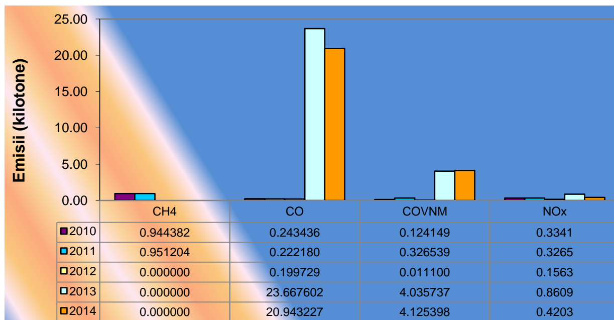
Fig. I.3.7. Evoluția emisiilor de precursori ai ozonului, din sectorul de activitate energie, în perioada 2010 - 2014
