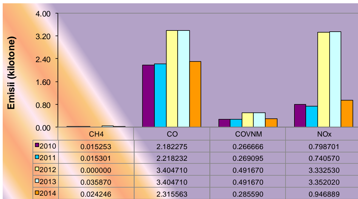
Fig. I.3.9. Evoluția emisiilor de precursori ai ozonului din transporturi, în perioada 2010 - 2014
