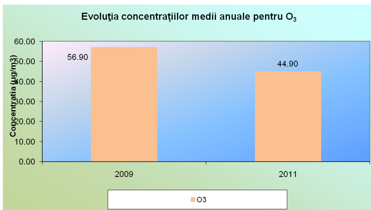
Fig. I.1.9. Evoluția concentrațiilor medii anuale pentru O 3
