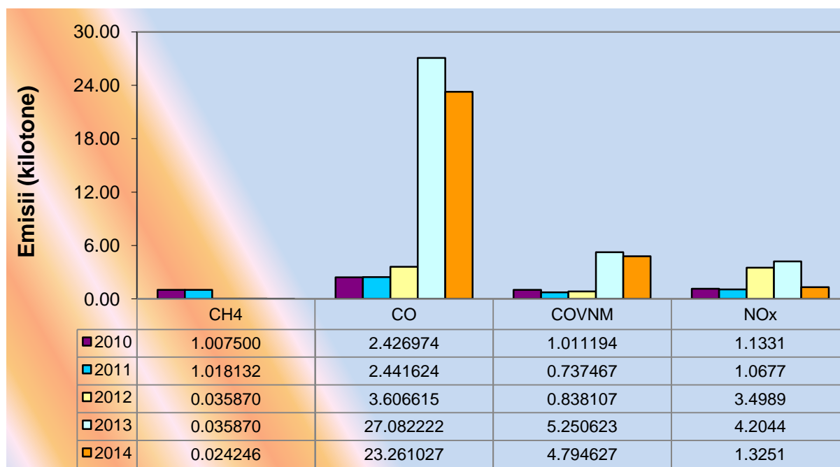
Fig. I.3.6. Evoluția emisiilor de precursori ai ozonului, în perioada 2010 - 2014
