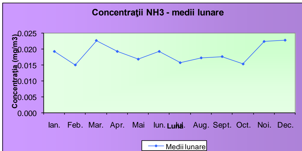
Fig. 8. Concentrații de NH 3 – medii lunare
