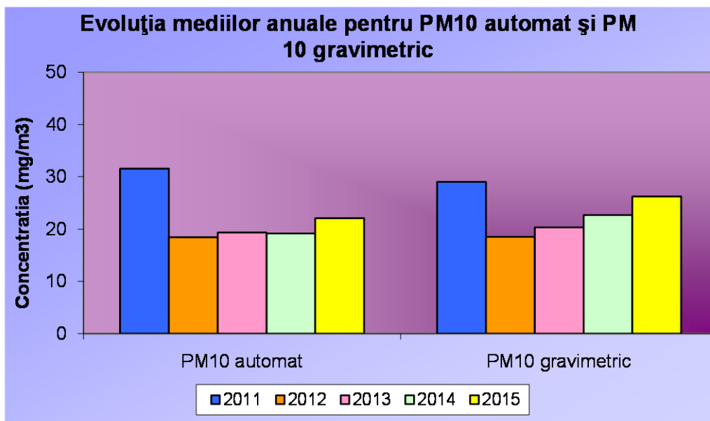
Fig. 12. Evoluția mediilor anuale pentru PM10 automat și PM10 gravimetric
