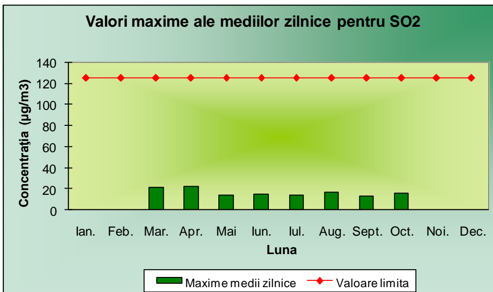
Fig. 4. Valorile maxime lunare ale mediilor zilnice pentru poluantul SO 2
