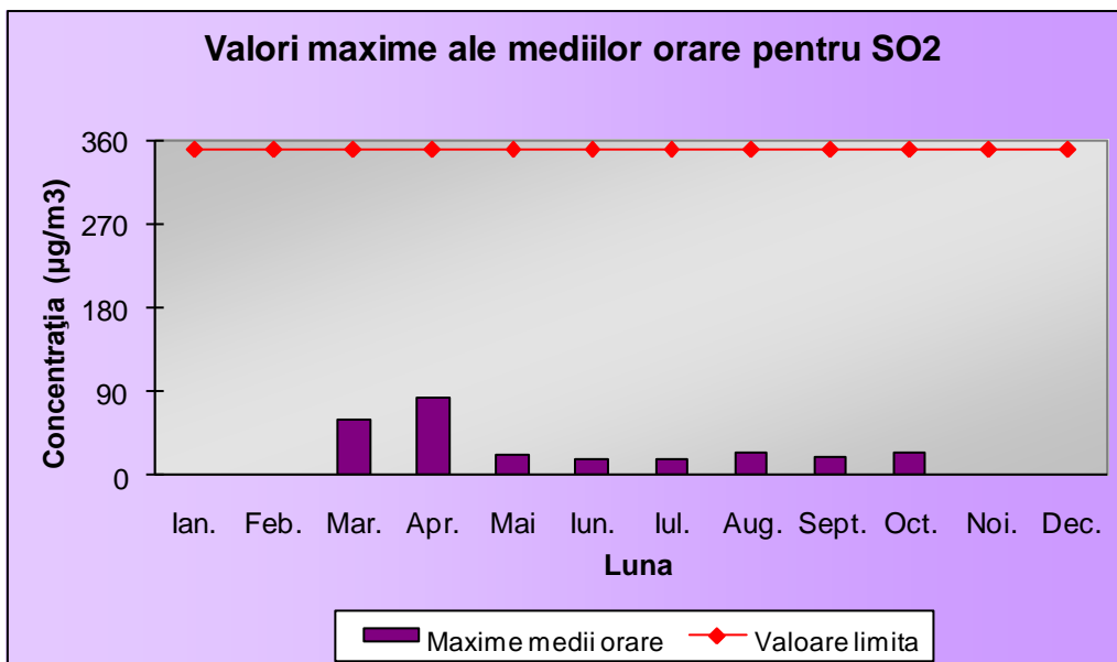
Fig. 3. Valorile maxime lunare ale mediilor orare pentru poluantul SO 2
