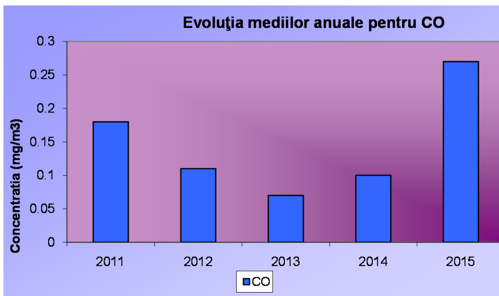
Fig. 11. Evoluția mediilor anuale pentru CO
