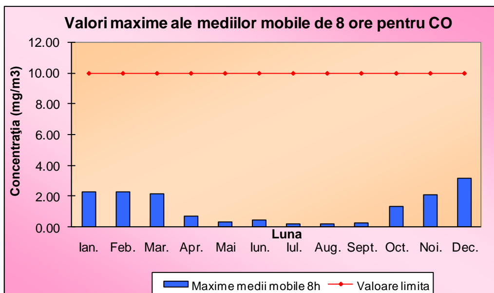
Fig. 7. Valorile maxime lunare ale mediilor mobile de 8 ore pentru poluantul CO
