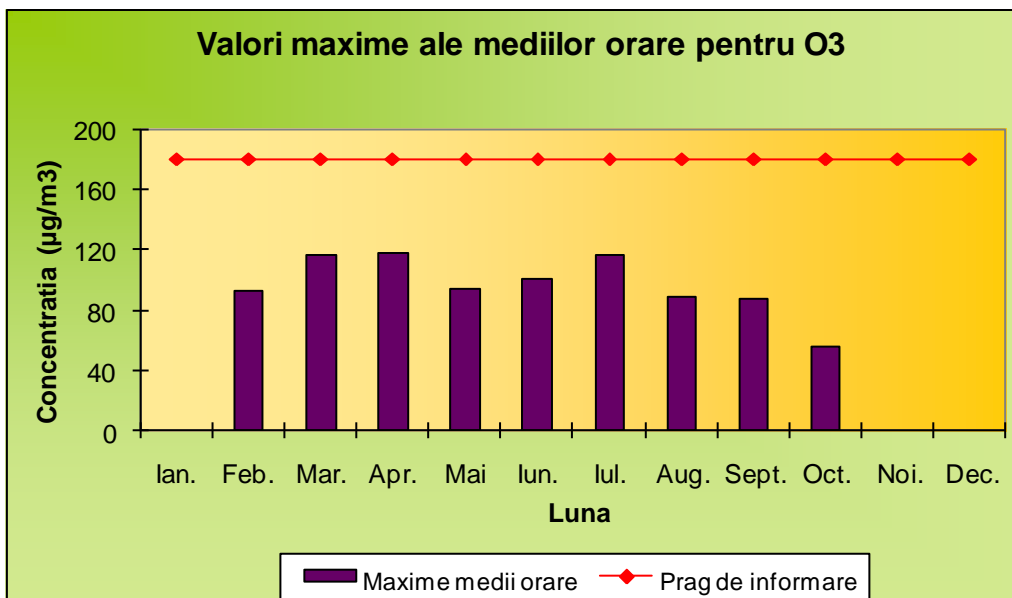
Fig. 9. Valorile maxime lunare ale mediilor orare pentru poluantul O 3
