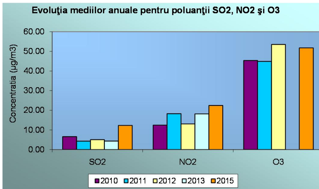
Fig. 10. Evoluția mediilor anuale pentru poluanții gazoși
