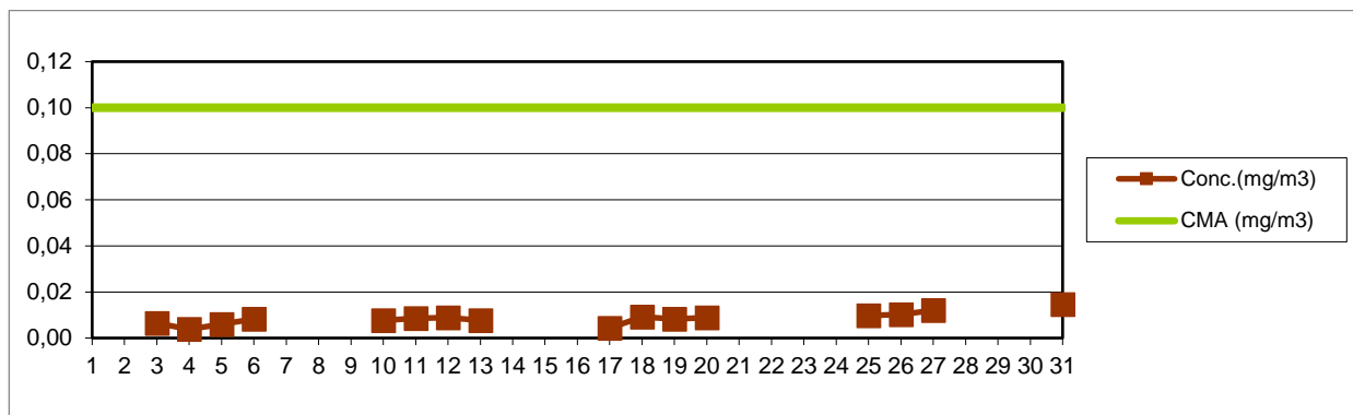
Fig. 1.11 Variația concentrațiilor medii zilnice ale indicatorului NH 3
