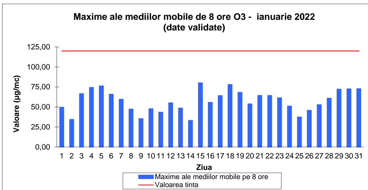
Fig 1.5 Maxime ale mediilor mobile de 8 h pentru indicatorul O3
