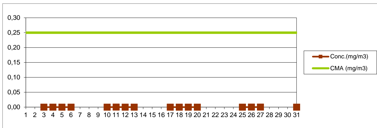
Fig. 1.9 Variația concentrațiilor medii zilnice ale indicatorului SO_2
