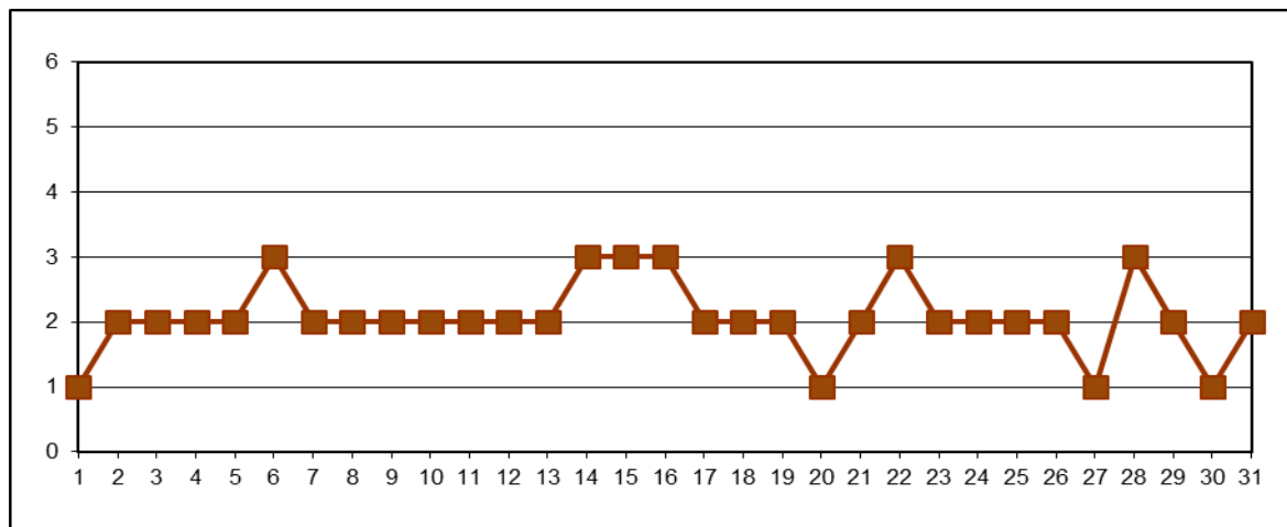
Fig.1.8 Evoluția indicelui general de calitate a aerului
