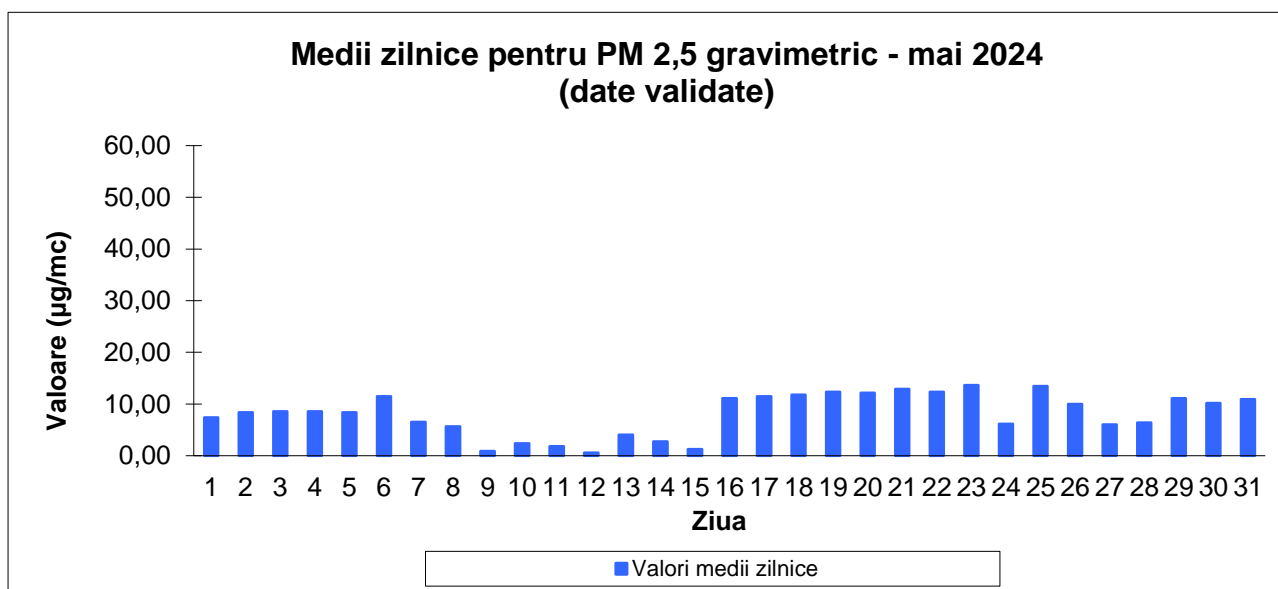
Fig 1.8 Mediile zilnice pentru indicatorul PM2,5
