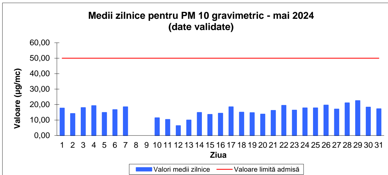
Fig 1.7 Mediile zilnice pentru indicatorul PM10
